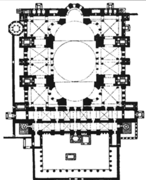
Κάτοψη τῆς Αγ. Σοφίας Κωνσταντινούπολης.
